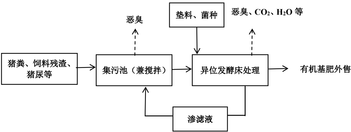
图 2.1.10-2 异位发酵床处理粪污工艺流程图
