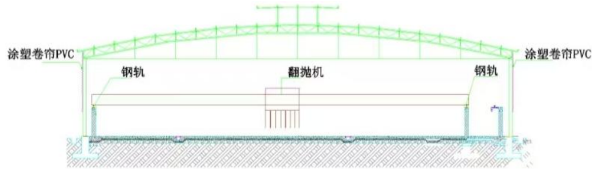
图 2.2.2.1-1 异位发酵床处理系统剖面图
