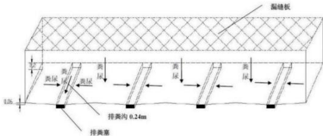
图 2.1.9-1 猪舍剖面图
