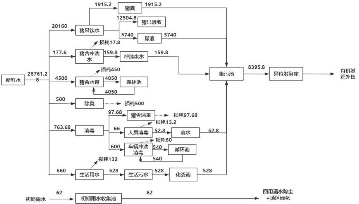
图 2.1.12.2-1 项目水平衡图 (m 3 /a)
