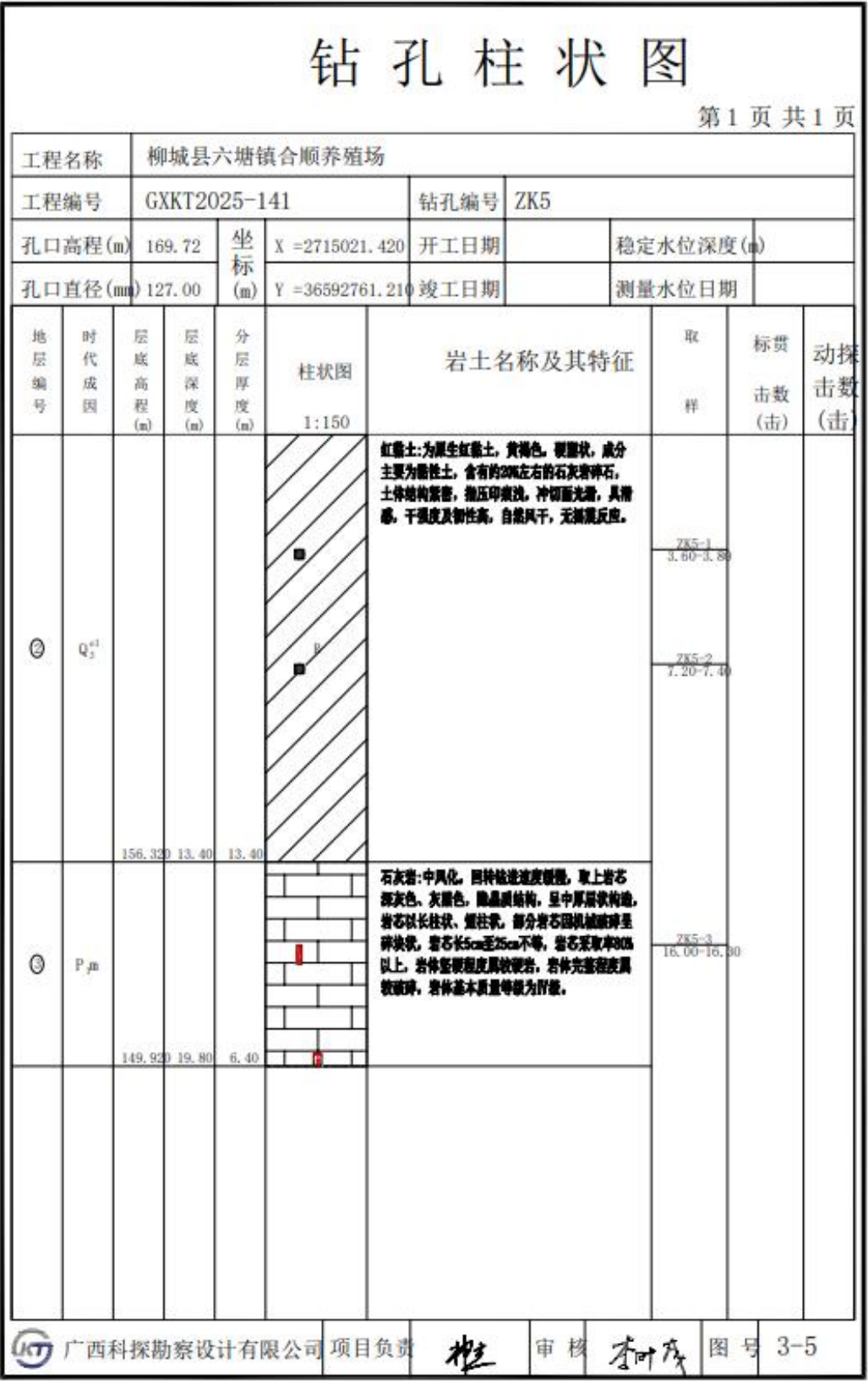
附图 30 ZK5 钻孔柱状图
