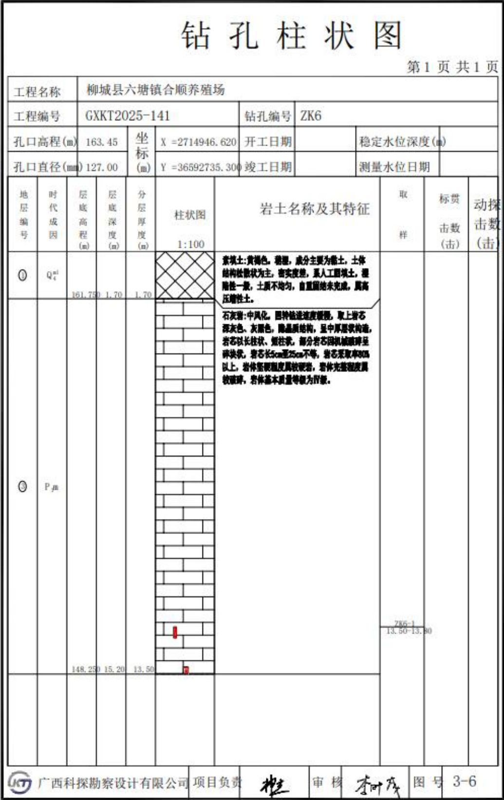
附图 31 ZK6 钻孔柱状图
