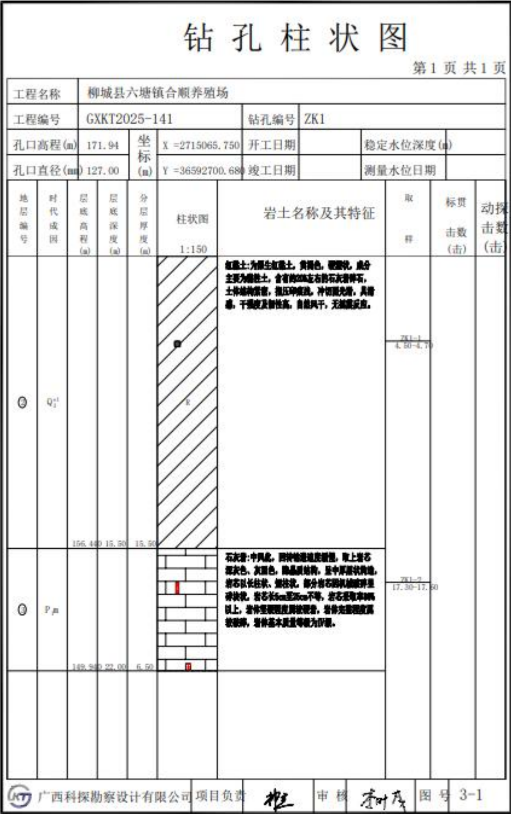
附图 26 ZK1 钻孔柱状图
