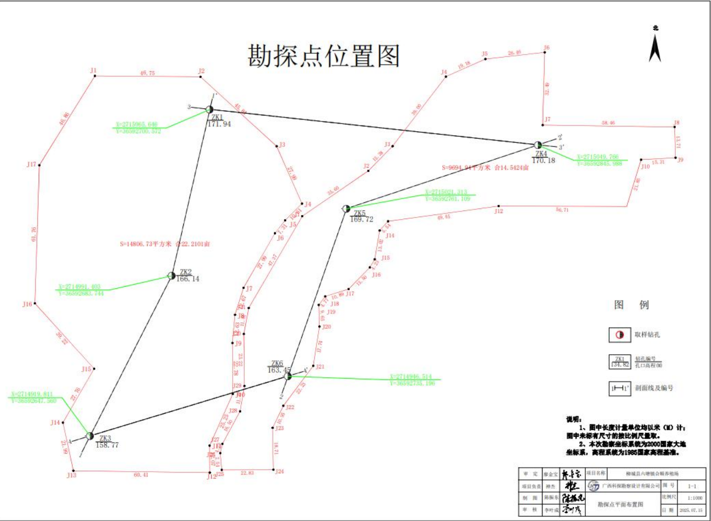
附图 25 地勘勘探点位置图
