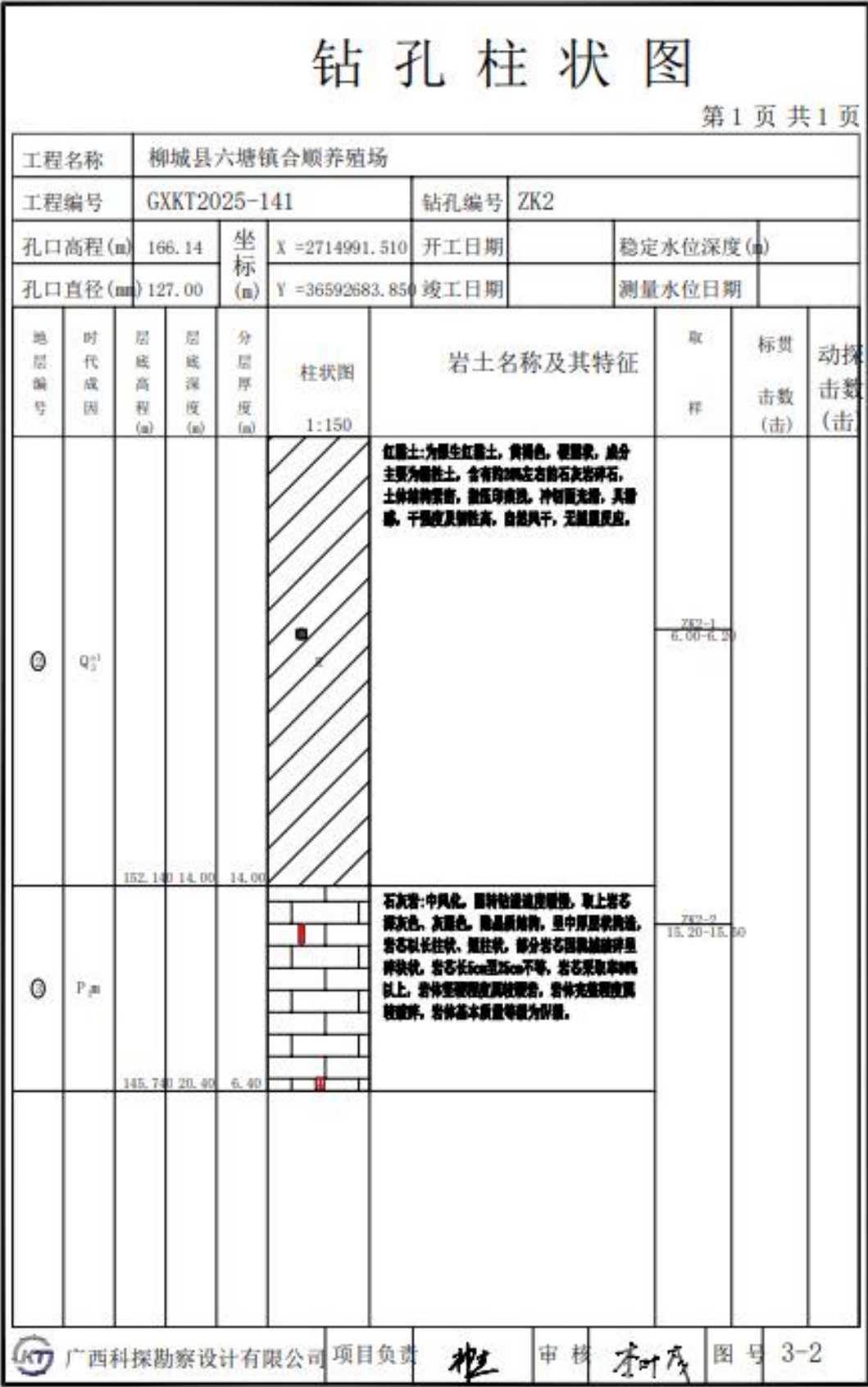
附图 27 ZK2 钻孔柱状图
