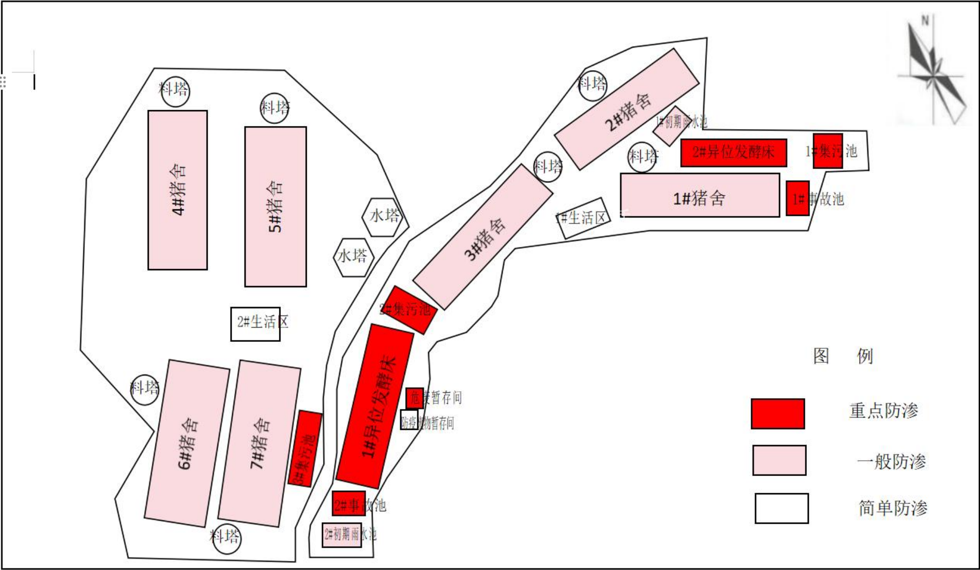
附图 7 项目分区防渗图
