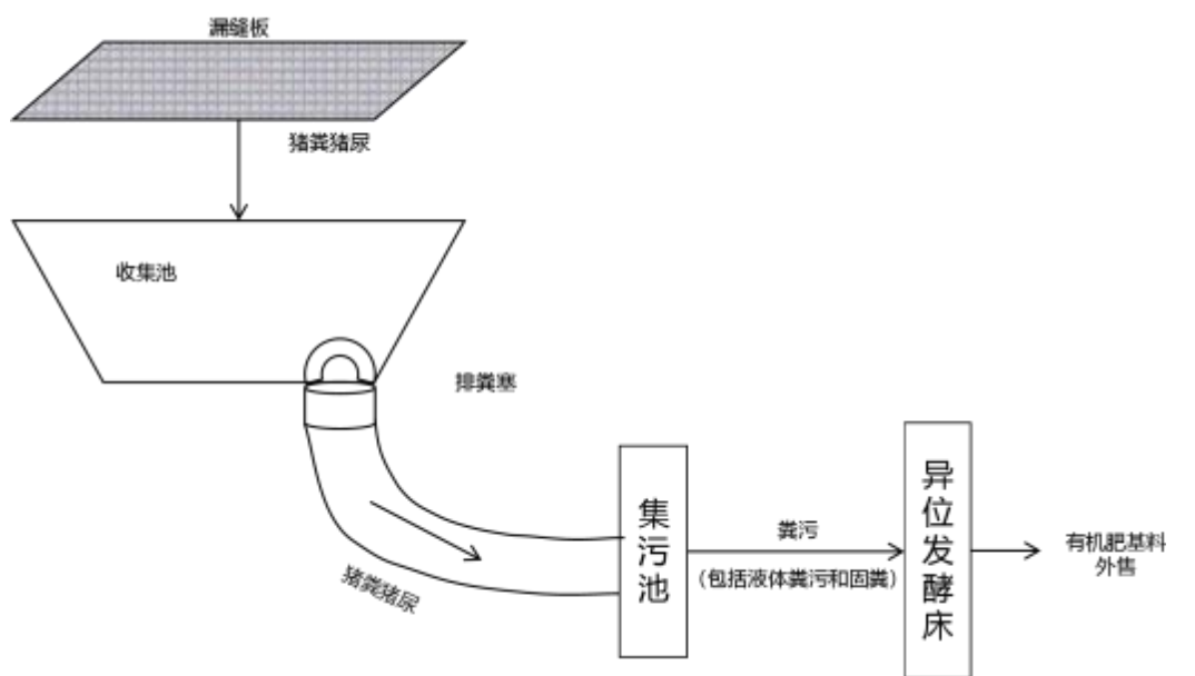
图 2.1.9-2 项目清粪工艺示图
