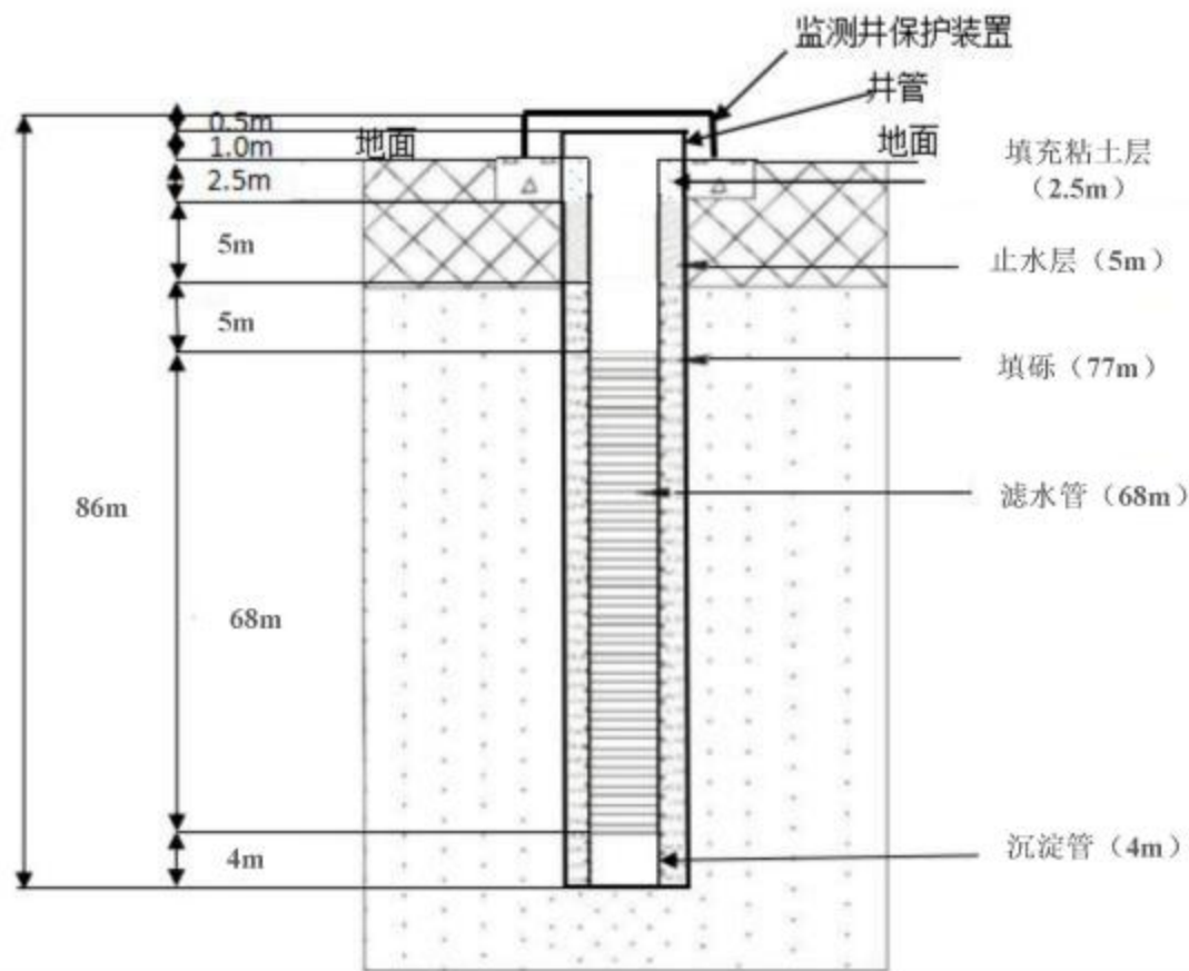
图 5.2.3.4-3 地下水环境监测井结构示意图
