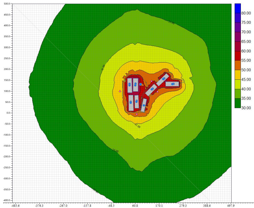
图 4.2.4.4-1 猪场昼间噪声预测
