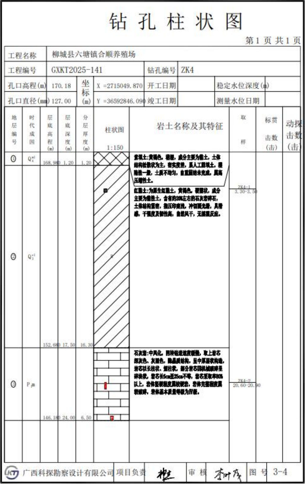
附图 29 ZK4 钻孔柱状图
