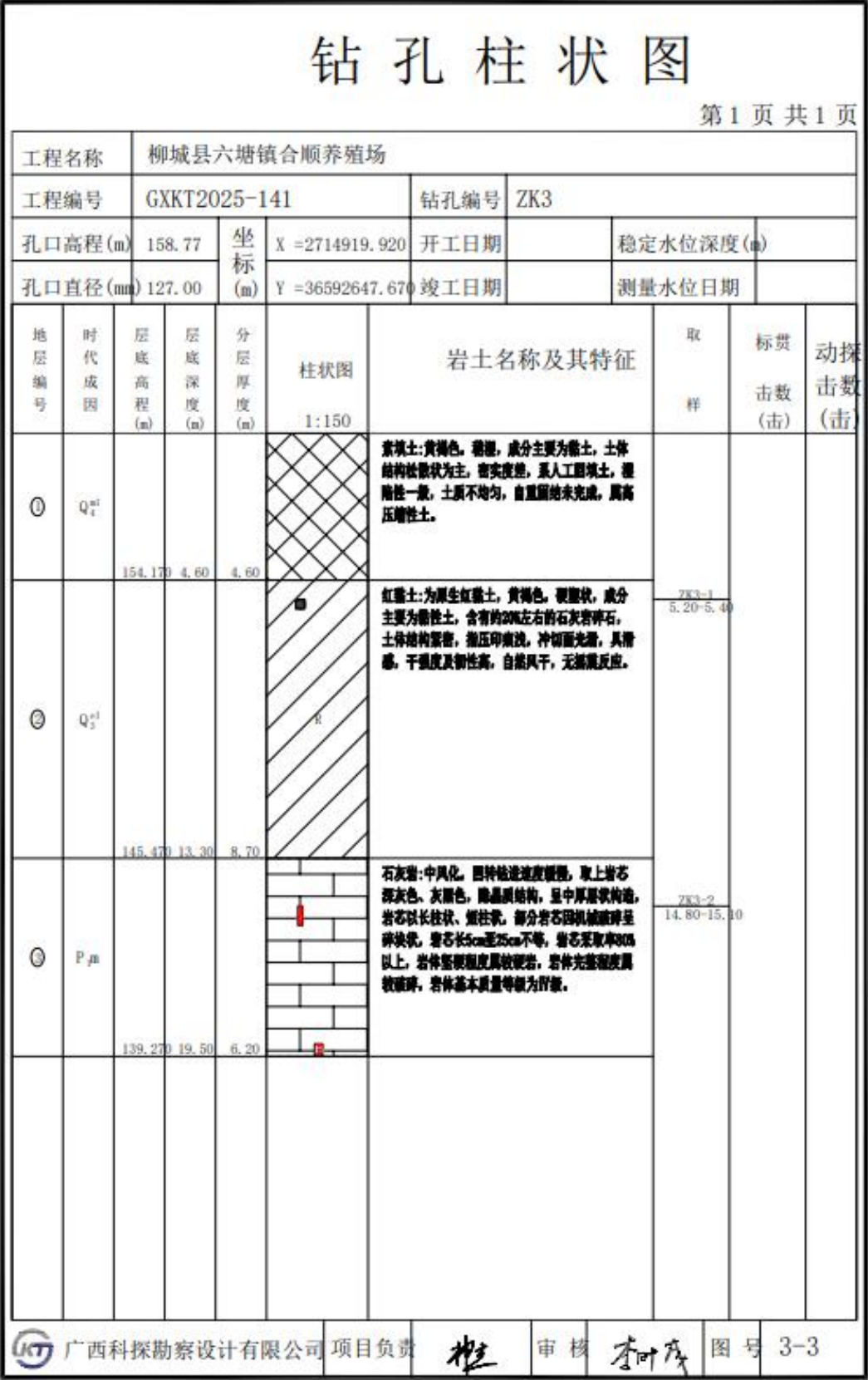
附图 28 ZK3 钻孔柱状图
