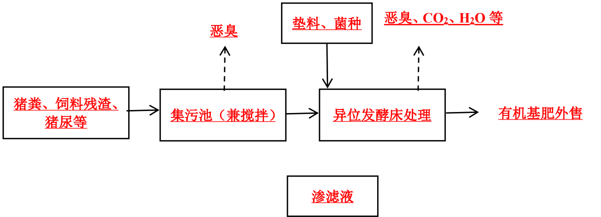
图 2.2.2.1-3 异位发酵床处理粪污工艺流程图
