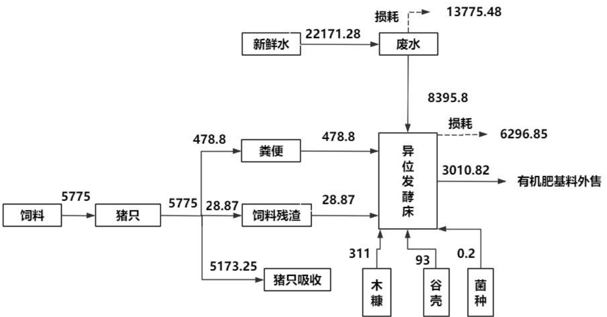
图 2.1.12.1-1 项目物料平衡图 (t/a)
